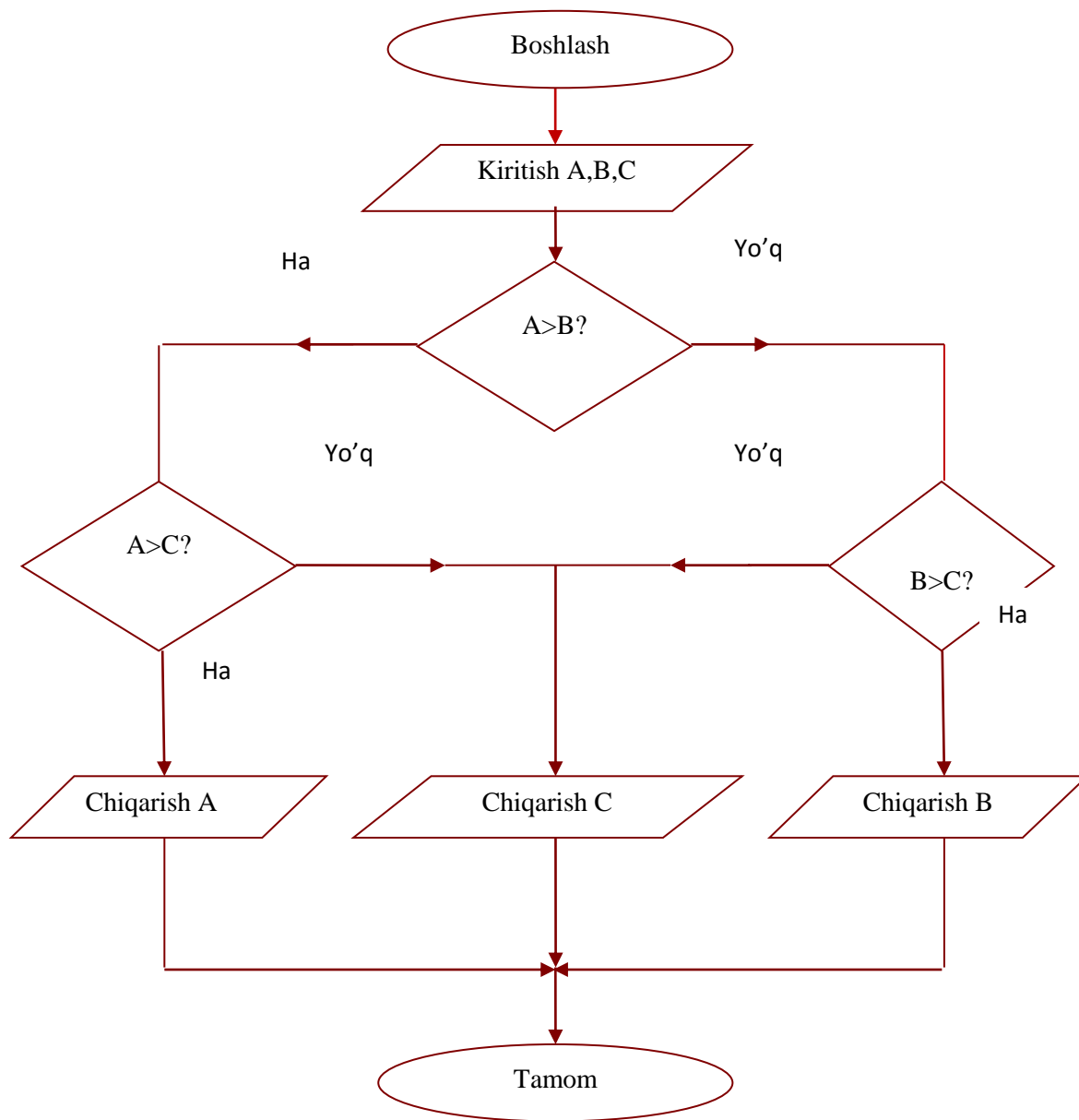
11.6-rasm. Uchta son ichidan eng kattasini topishni boshqa versiyasi.
