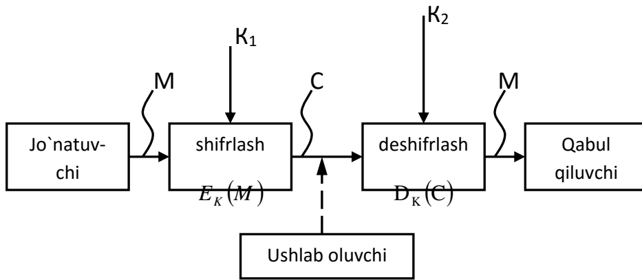
21.2-rasm. Ochiq kalitli asimmetrik kriptotizimning umumlashma sxemasi.
