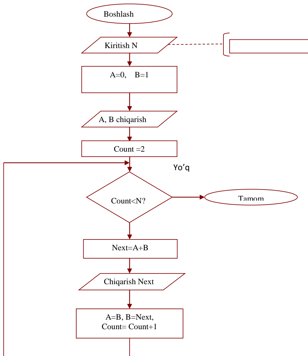
11.12-rasm. Fibonachi ketma-ketligidagi sonlarni chiqarish algoritmi.
