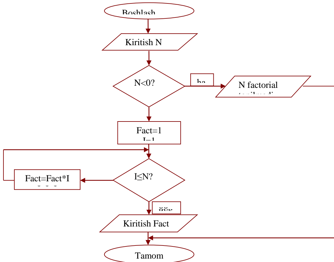
11.11-rasm. Sonlarni faktorialini aniqlash algoritmi 43 .
