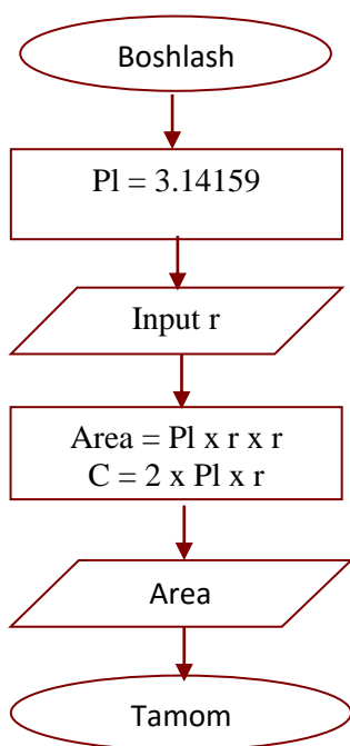
11.2-rasm. R radiusga ega aylananing uzinasini va yuzini topish blok chizmasi.
