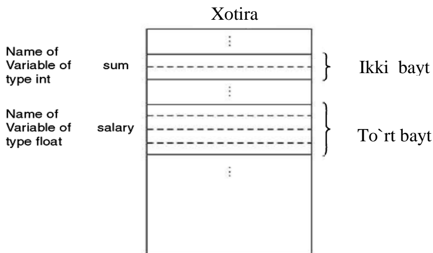
12.8-rasm. Xotiradagi int va float turidagi o`zgaruvchilar
