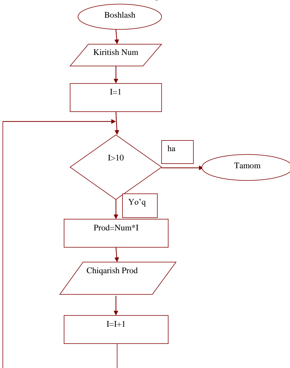
11.9-rasm. Sonlarni ko`paytirish jadvalini chiqarish algoritmi
