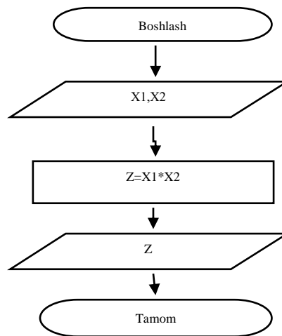
10.6-rasm. Ikkita sonni ko`paytirish algoritmi
