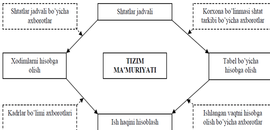
20.7-rasm. Kadrlni boshqarishni ta`minlash uchun kompleks axborot tizimi modullarining funksional chizmasi
