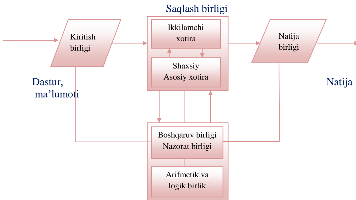
3.3-rasm. Kompyuter sistemasining blok rasmi 2
