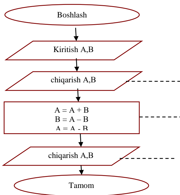
11.4- rasm. Ikkita sonning vaqtinchalik o'zgaruvchidan foydalanmay joyini almashtirish.
