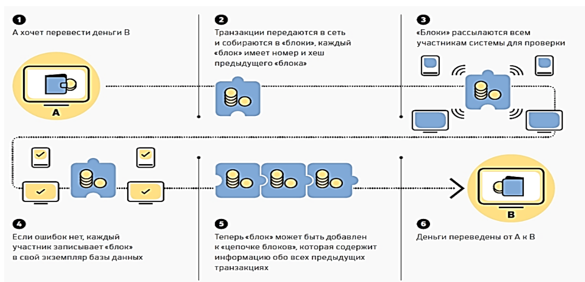
13.2-rasm. Kripto valyuta misolida blokirovka qilish tamoyili 137
