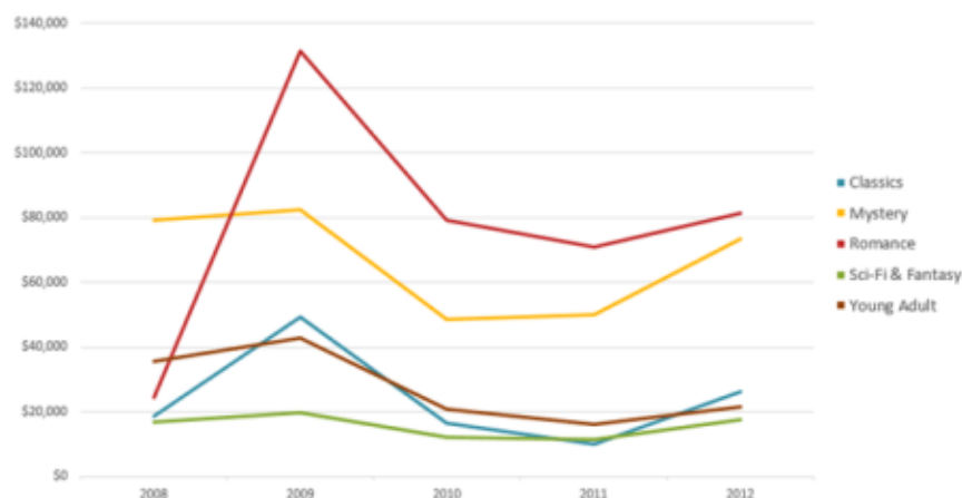
5.73-rasm. Grafik.
