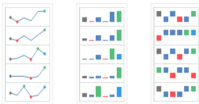
5.84. Sparklayn turlari.
