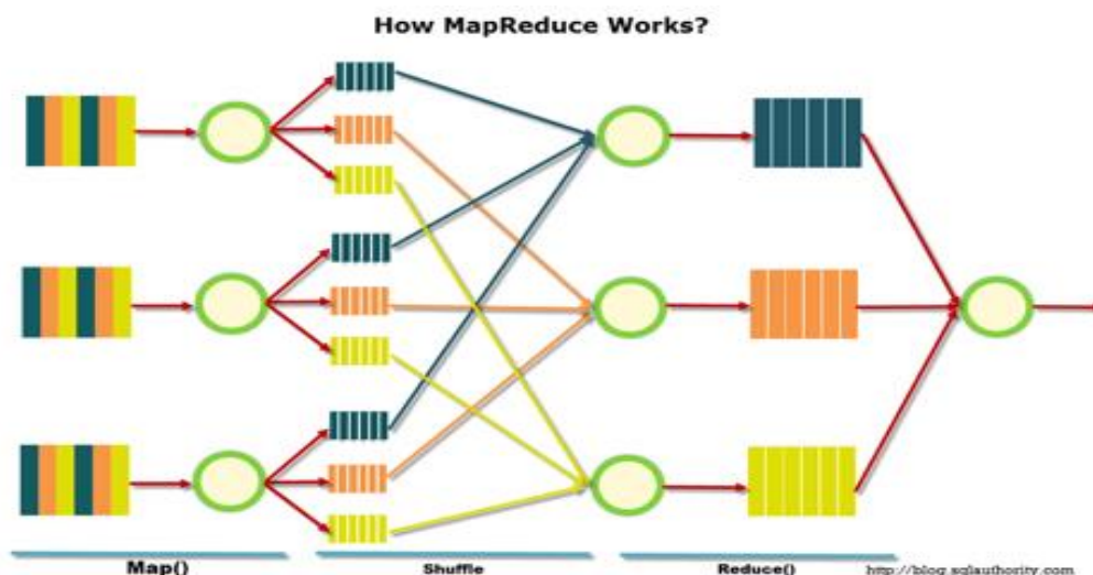
Рис. 8.4. MapReduce.
