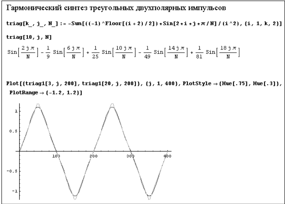
Рис. 6.5. Гармонический синтез симметричных треугольных импульсов
