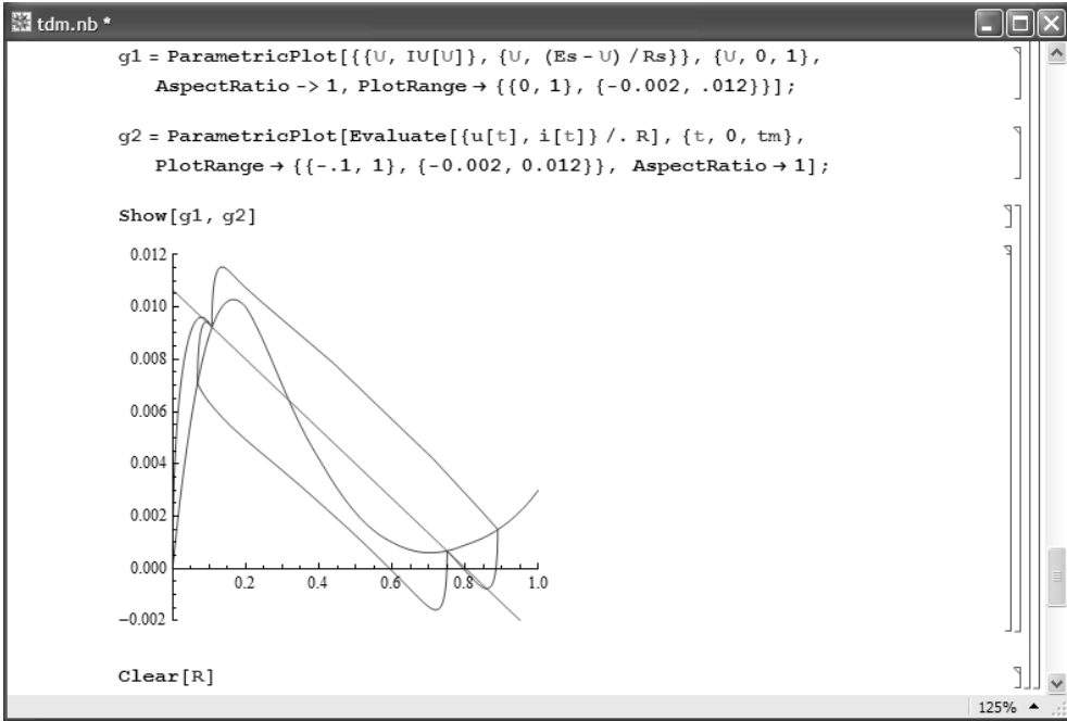
Рис. 10.44. Фазовый портрет колебаний в схеме триггера на туннельном диоде
