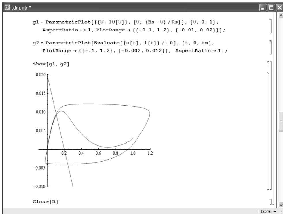
Рис. 10.42. Фазовый портрет одного цикла колебаний ждущего релаксатора
