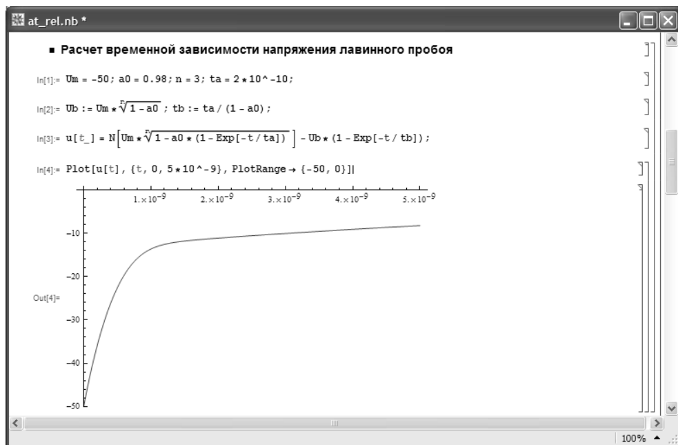
Рис. 10.35. Расчет спада напряжения на коллекторе лавинного транзистора при его включении – динамического пробоя
