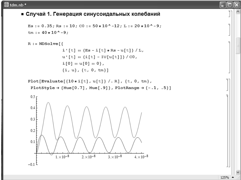
Рис. 10.39. Расчет временной зависимости напряжения u(t) и тока i(t) для случая 1
