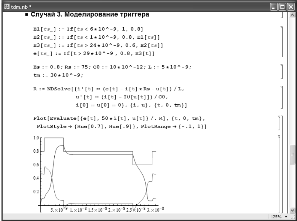
Рис. 10.43. Задание временной зависимости e(t) и получение временных зависимостей импульсов при работе цепи с туннельным диодом в триггерном режиме
