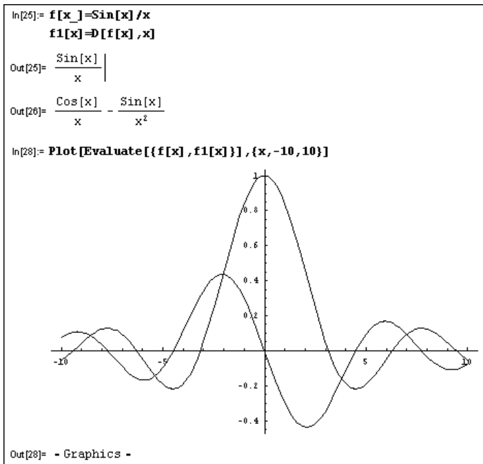
Рис. 5.1. График функции \text{Sin}[x]/x и ее производной
