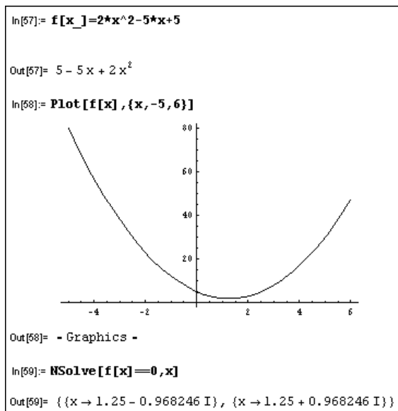
Рис. 5.21. Иллюстрация решения квадратного уравнения для случая двух комплексных корней
