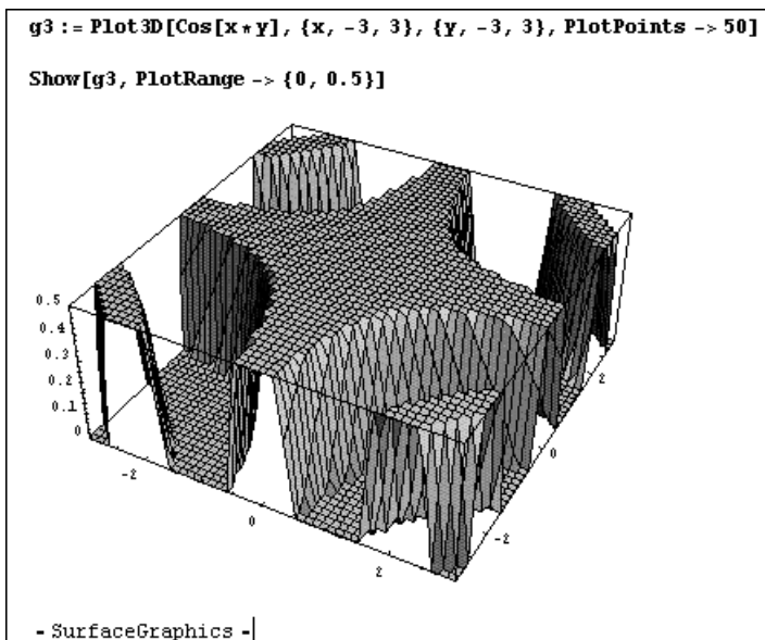
Рис. 8.21. Математическая поверхность с отсеченной верхней частью
