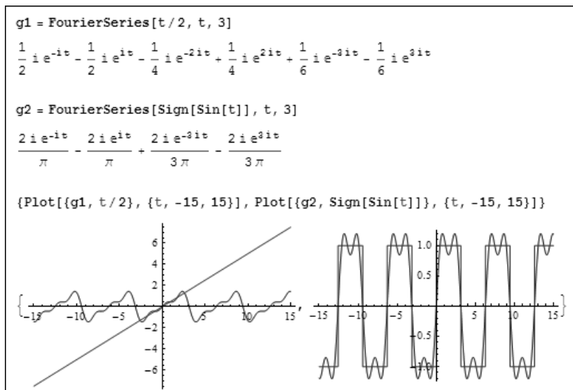
Рис. 10.24. Примеры разложения в ряд Фурье линейно нарастающей функции и меандра
