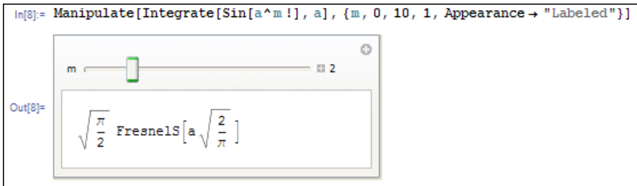
Рис. 1.31. Вычисление интеграла с подынтегральной функцией \sin(a^m!) – случай m=2
