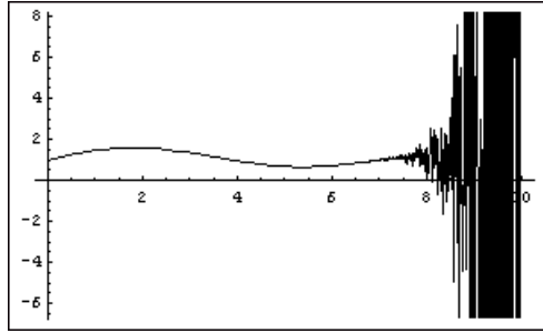
Рис. 6.10. График полинома степени 40, иллюстрирующий возникновение числовой неустойчивости в правой части, при больших x
