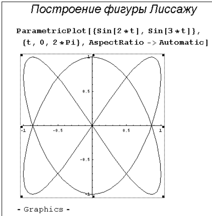
Рис. 8.12. Построение фигуры Лиссажу
