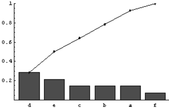
Рис. 6.55. Пример построения диаграммы Парето
