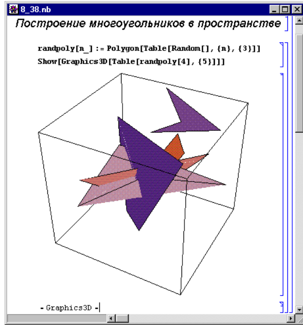
Рис. 8.38. Построение в пространстве взаимно пересекающихся плоских многоугольников
