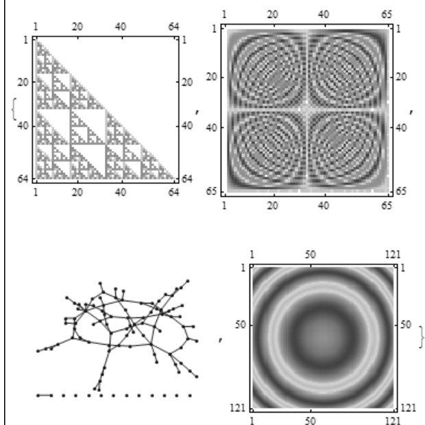
Рис. 10.21. Примеры применения функции визуализации матриц MatrixPlot
