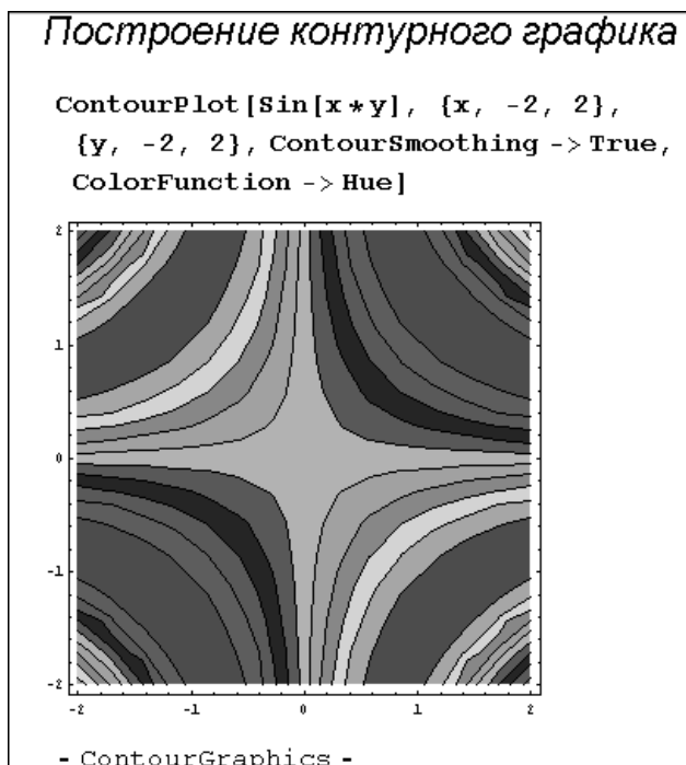
Рис. 8.15. Контурный график поверхности \sin(x \cdot y) с закраской областей между линиями равного уровня оттенками серого цвета
