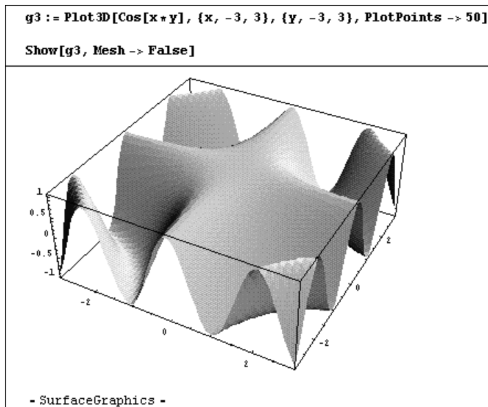
Рис. 8.24. Математическая поверхность с удаленными линиями каркаса
