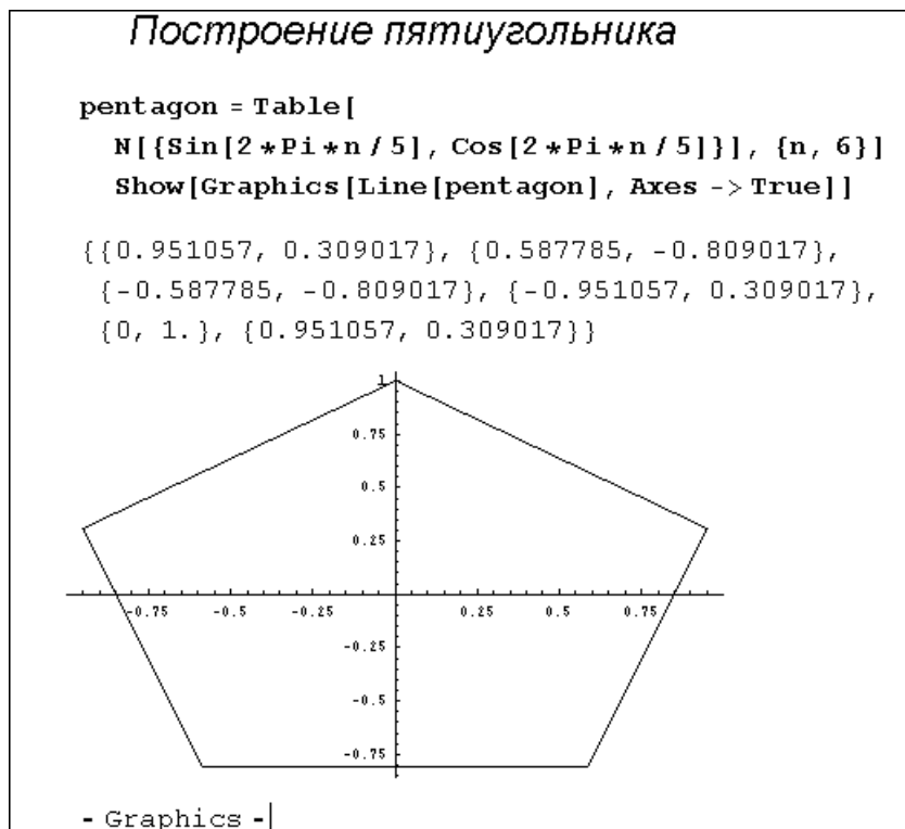
Рис. 8.11. Построение пятиугольника
