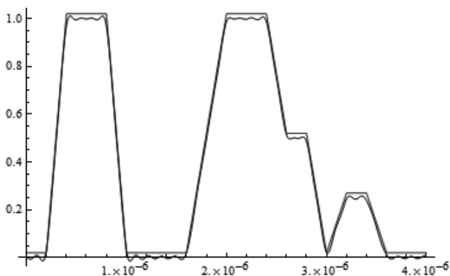
Рис. 10.45. График сигнала y[t] и его представления рядом Фурье
