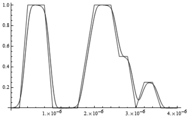
Рис. 10.47. Сигнал на входе и на выходе фильтра
