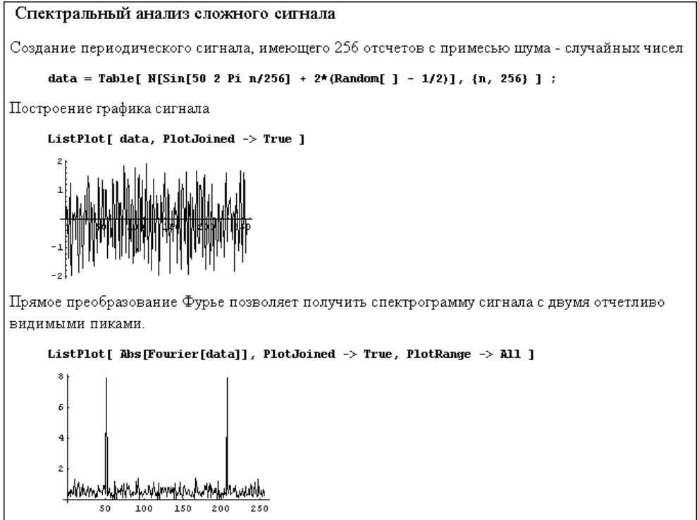
Рис. 6.33. Получение спектра сложного сигнала с помощью прямого преобразования Фурье
