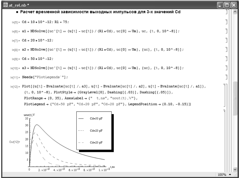
Рис. 10.36. Расчет временной зависимости выходных импульсов
