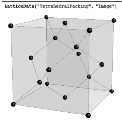
Рис. 10.14. Пример построения рисунка решетки
