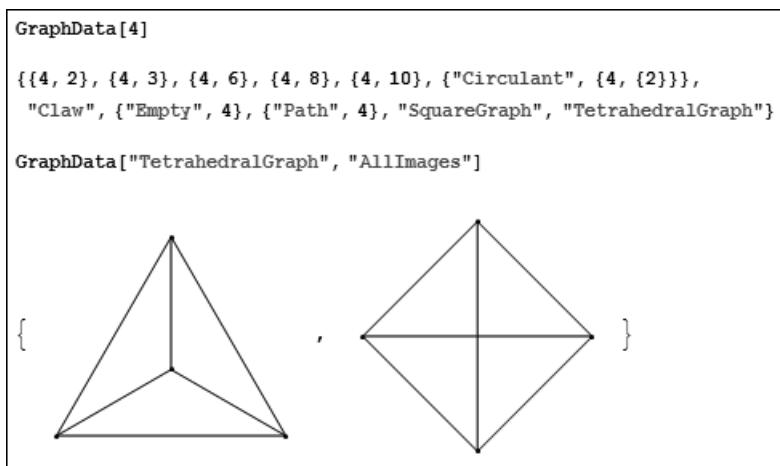
Рис. 10.12. Простые примеры применения функции GraphData
