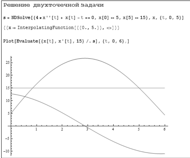
Рис. 10.28. Пример решения дифференциального уравнения второго порядка с двумя граничными условиями
