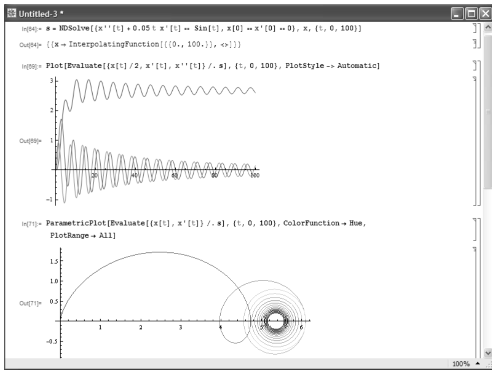
Рис. 10.29. Пример решения дифференциального уравнения второго порядка с построением цветного (в оригинале) фазового портрета
