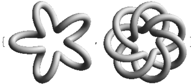
Рис. 10.13. Построение графиков двух узлов
