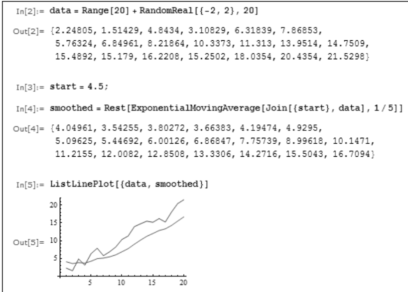
Рис. 6.58. Пример сглаживания 20 точек с графической визуализацией
