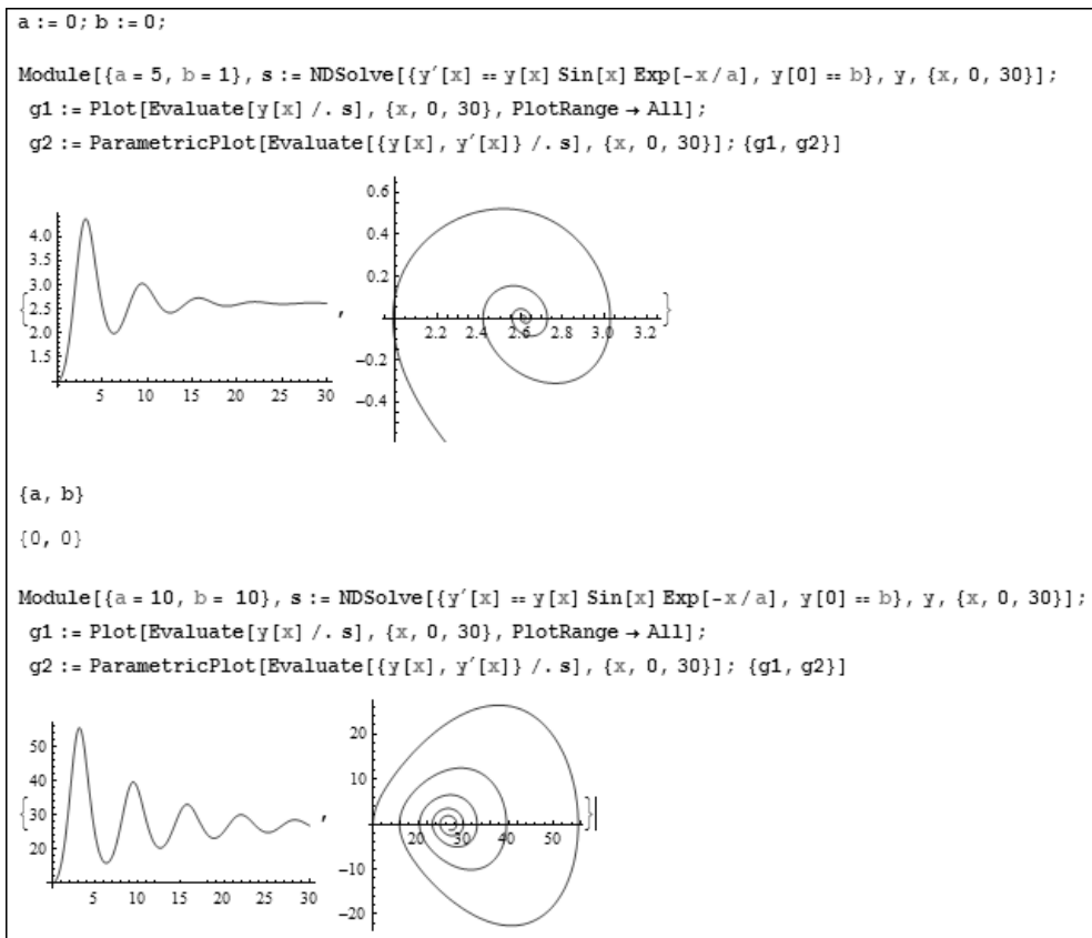
Рис. 10.26. Пример решения дифференциального уравнения, оформленного в виде модуля
