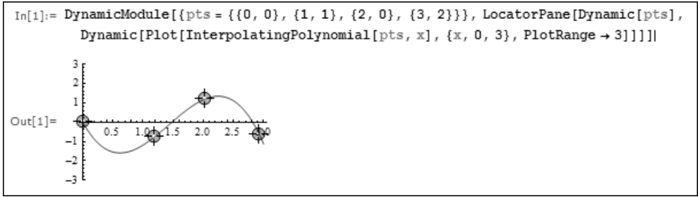
Рис. 8.52. Иллюстрация полиномиальной аппроксимации для четырех точек
