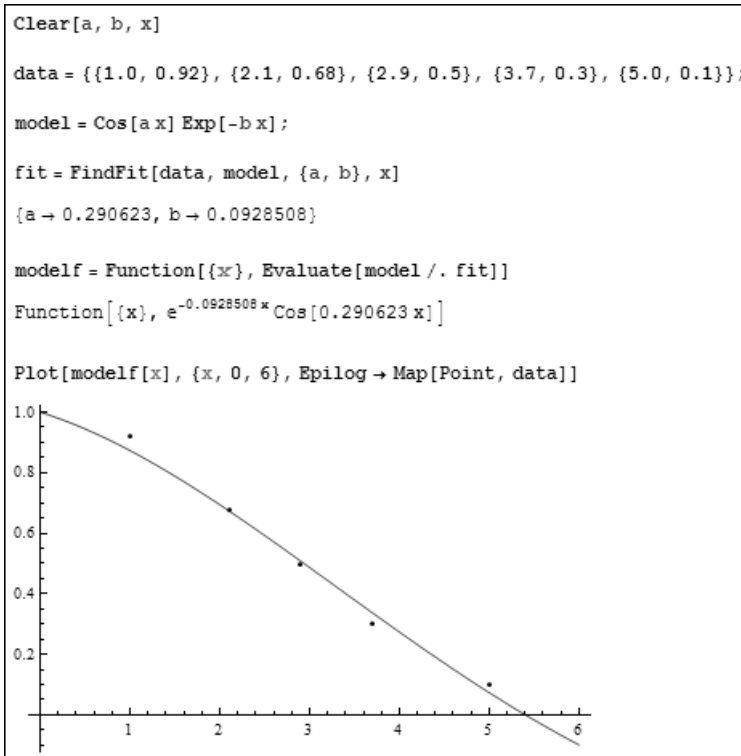
Рис. 6.40. Пример выполнения нелинейной регрессии
