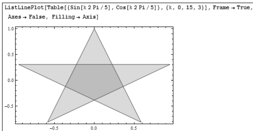
Рис. 8.55. Построение звезды
