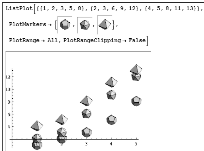
Рис. 8.94. Пример обозначения точек графиков трехмерными фигурами
