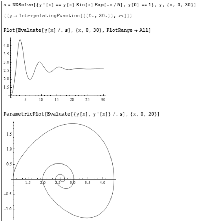
Рис. 10.25. Пример решения дифференциального уравнения первого порядка и вывода графиков решения в форме зависимости y(x) и фазового портрета
