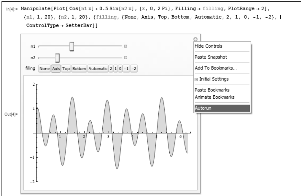
Рис. 8.50. Модуль, иллюстрирующий построение графика суммы двух гармонических колебаний с изменяемой кратностью частот и различные виды закрашки графика с помощью меню
