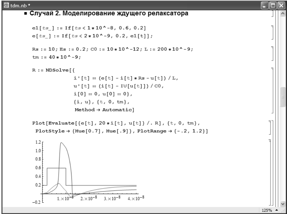
Рис. 10.41. Моделирование ждущего релаксатора
